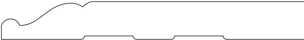
KL 299 .687 x 5.500
