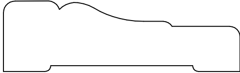
KL 104 .750 x 2.500
