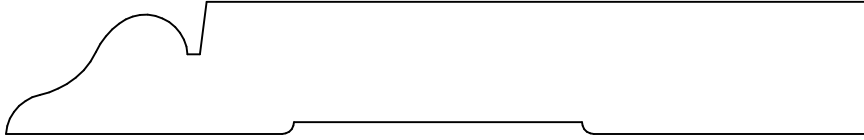
KL 215 .687 x 4.500
