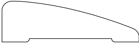
KL 102 .750 x 2.500
