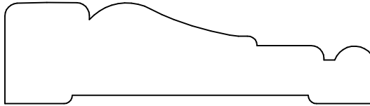
KL 105 .750 x 2.750
