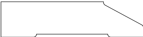
KL 6219 .750 x 3.000
