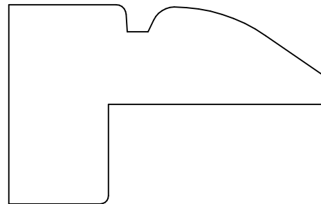
KL 11260 1.500 x 2.375
