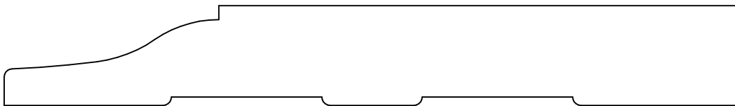
KL 14229 .750 x 5.500
