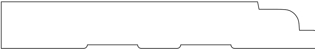
KL 4272 .812 x 5.500
