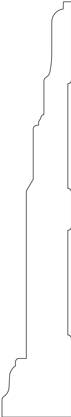
KL 6248 1.250 x 7.437
